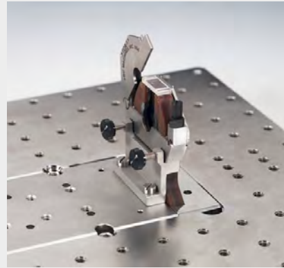
Modelo 4-500 equipado con utillaje (estrecho) del cabezal AMI Modelo 9-500TCA.
